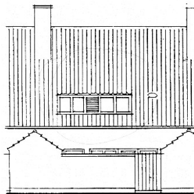
FACADE MOD ØST
